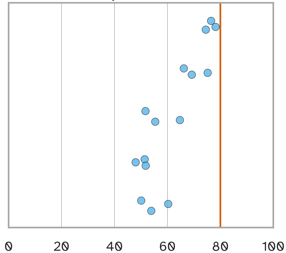
Exponencial
